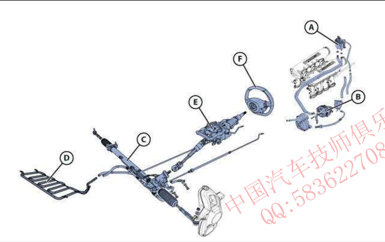
转向系统布置
